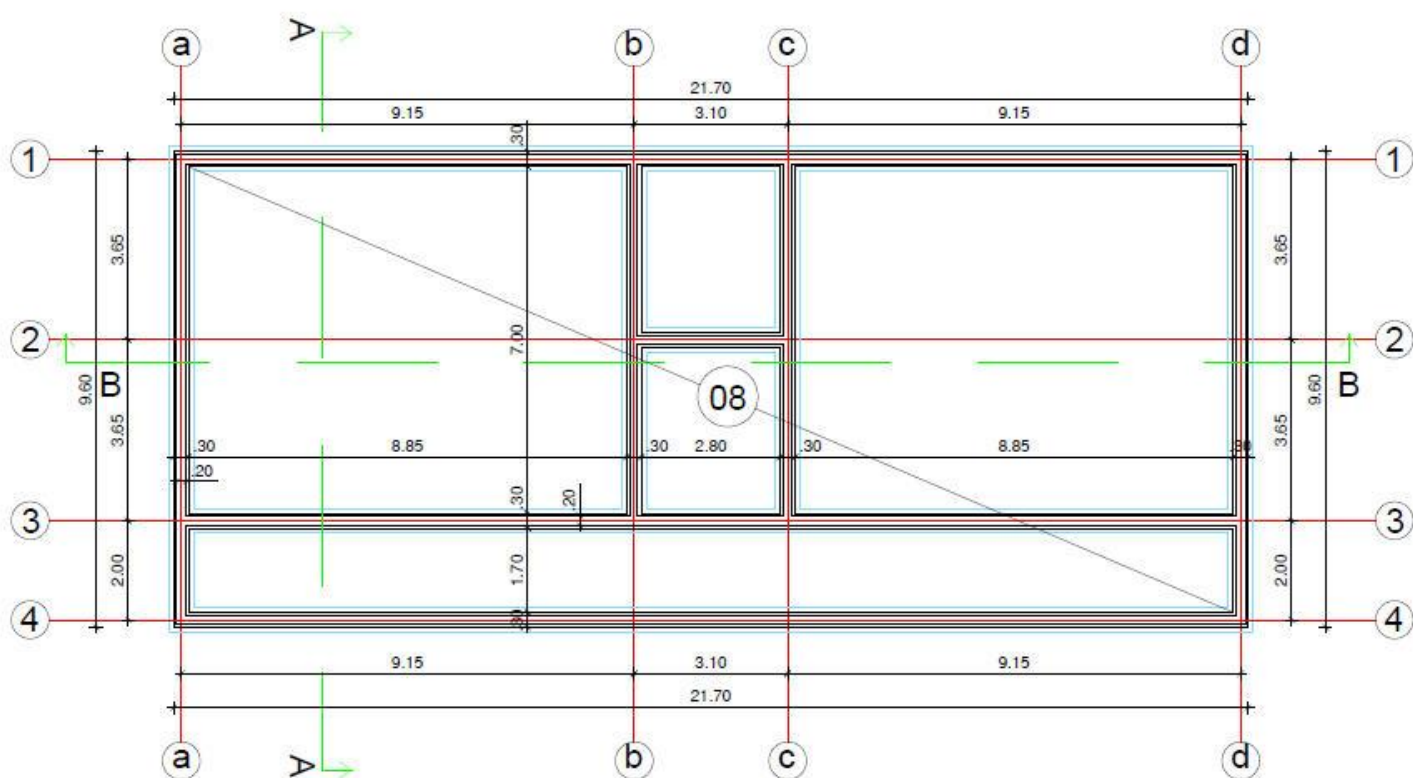
Plan de Fondation
