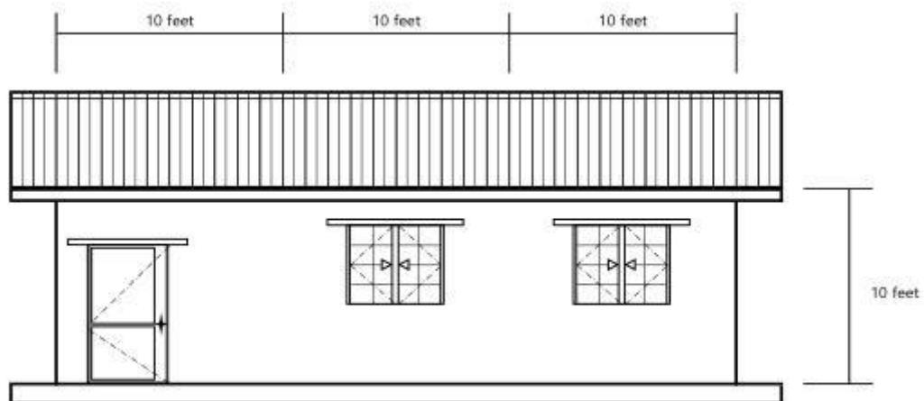
그림2) 입면도
