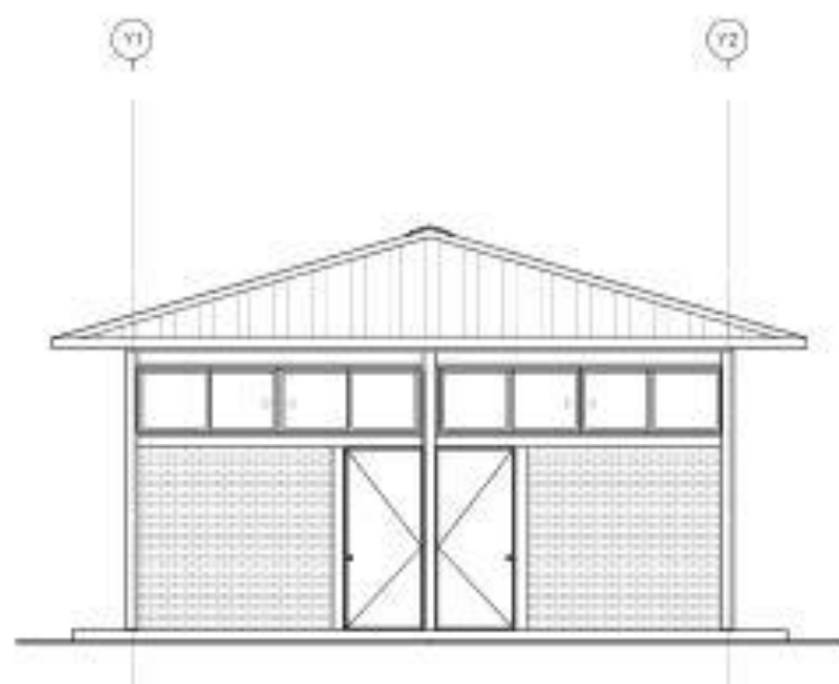
2 측면도 축척: 1 / 120
