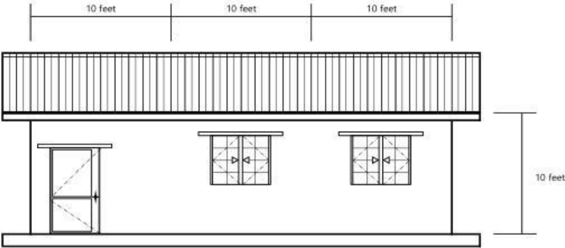
그림2) 입면도
