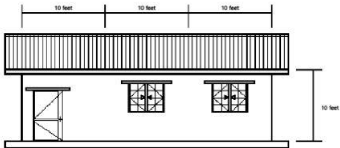
그림2) 입면도
