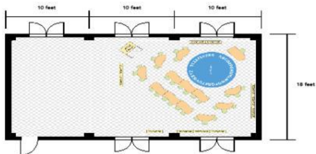
그림1) 평면도
