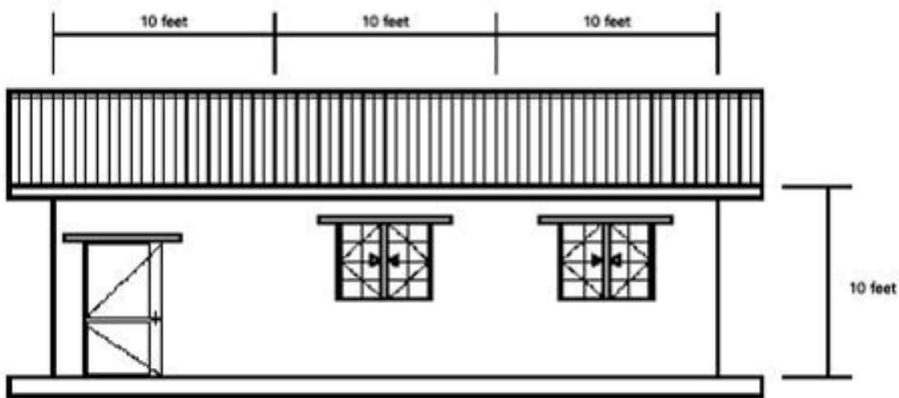
그림 2) 입면도
