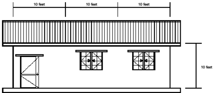
그림2) 입면도
